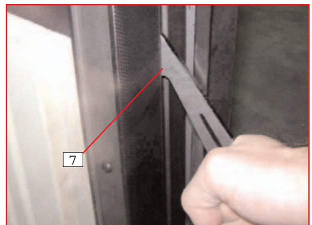
Figura 4 : bloqueo puerta cerrada (rotar el gatillo unos 90°)
